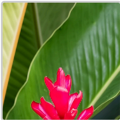
AHD: 32.8 dB
