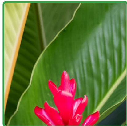
MLRI: 36.5 dB
